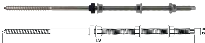
VFX - Viti per fotovoltaico inox A2
